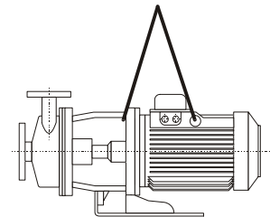
Fig.1 Transporte
