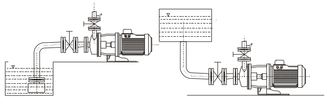
Bild 2 Rohrleitungenanschluss
